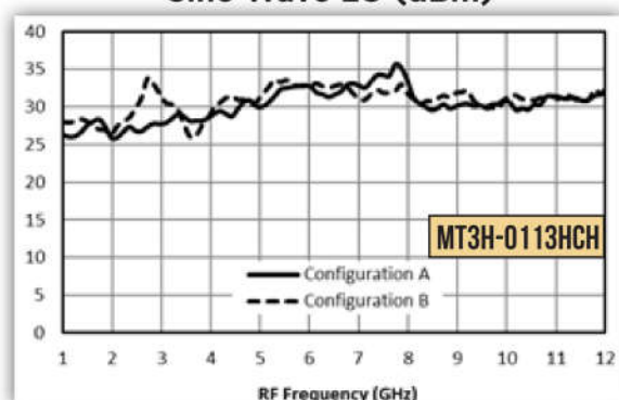
Input IP3: +20dBm Sine Wave LO (dBm)
